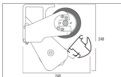
Diagramma di copertura a parete / soffitto Wall/Ceiling covering diagram
