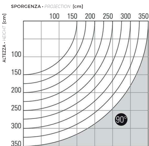
Diagramma di copertura a parete / soffitto Wall/Ceiling covering diagram
