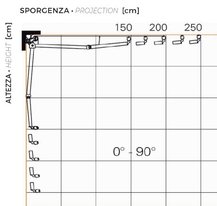
Diagramma di copertura a parete / soffitto Wall/Ceiling covering diagram
