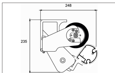
Ingombri installazi. parete/soffitto Installation dimension wall/ceiling
