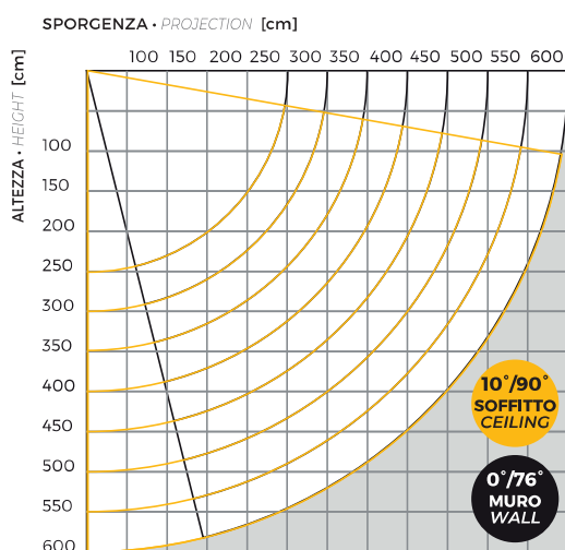
Diagramma di copertura Covering diagram
