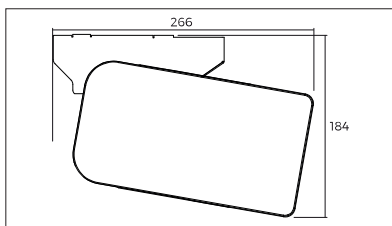
Montaggio a soffitto Ceiling installation
